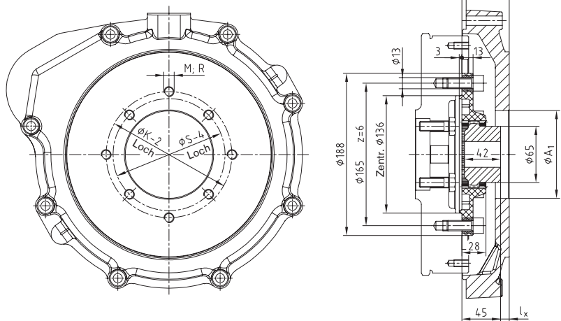
BoWex® 48 FLE-PA Ø 188 / Pumpenanbaugehäuse
