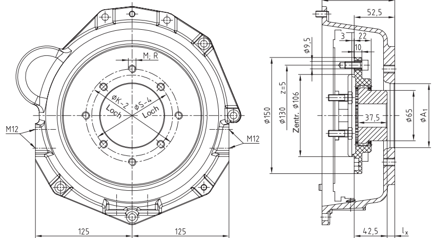
BoWex® 48 FLE-PA Ø 150 / Pumpenanbaugehäuse
