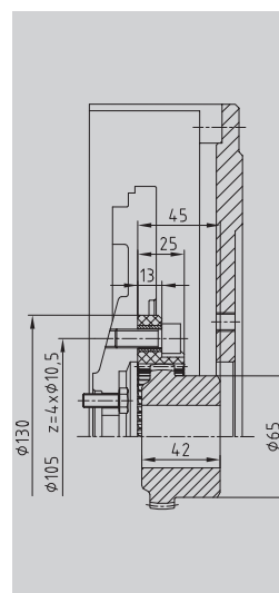
BoWex® 48 FLE-PA, Ø130 Mitsubishi L-Serie / K-Serie
