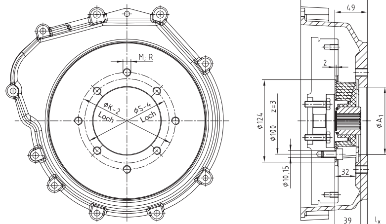
MONOLASTIC® 28 Ø 124 / Pumpenanbaugehäuse
