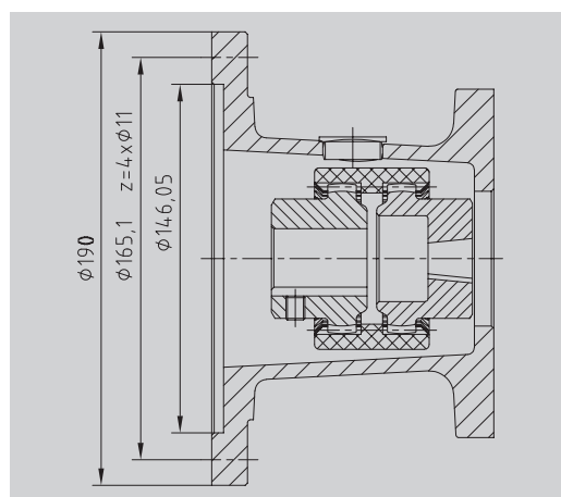
BoWex® Wellenkupplung Bauart M28 und M32 Gehäuseanschluss nach SAE J609A
