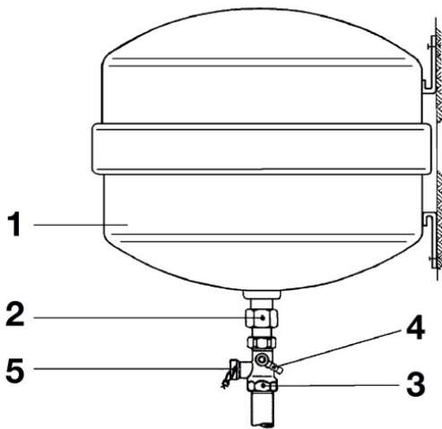
Kappenventil mit Außdehnungsgefäß
