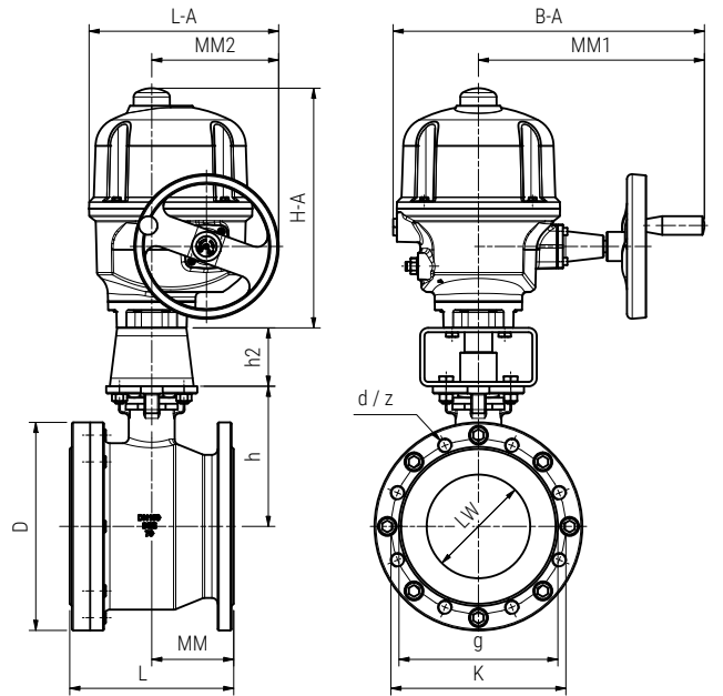
DN125 / DN150: Kugelhahn auf Rohrleitung mit Sackloch Tiefe 22mm / 25mm DN125 / DN150: Ball valve on pipe by blind hole depth 22mm / 25mm
