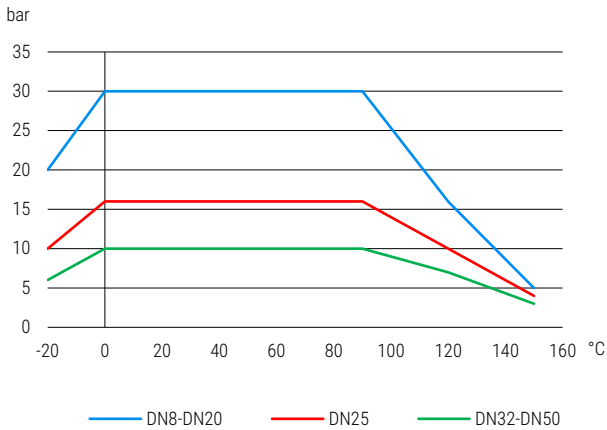
Druck-Temperatur-Diagramm pressure-temperature-diagram
