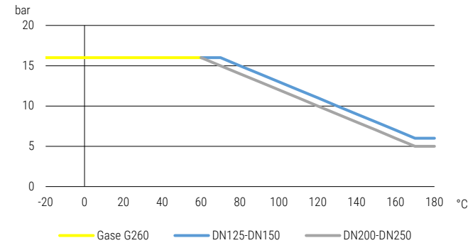
Druck-Temperatur-Diagramm pressure-temperature-diagram
