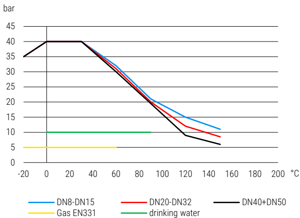
Druck-Temperatur-Diagramm pressure-temperature-diagram
