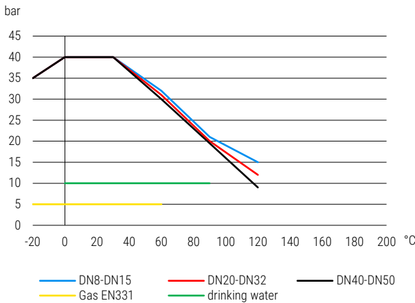
Druck-Temperatur-Diagramm pressure-temperature-diagram
