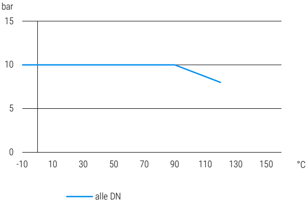
Druck-Temperatur-Diagramm pressure-temperature-diagram
