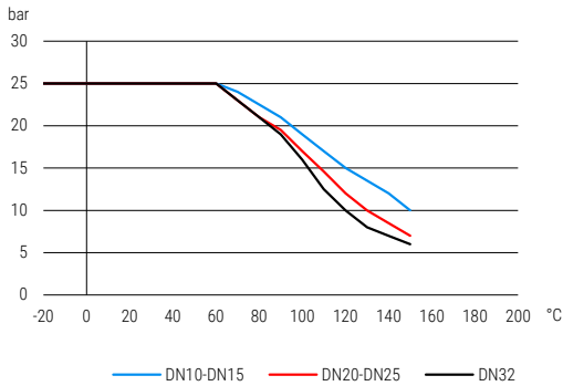
Druck-Temperatur-Diagramm pressure-temperature-diagram
