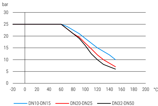
Druck-Temperatur-Diagramm pressure-temperature-diagram
