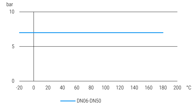
Druck-Temperatur-Diagramm pressure-temperature-diagram
